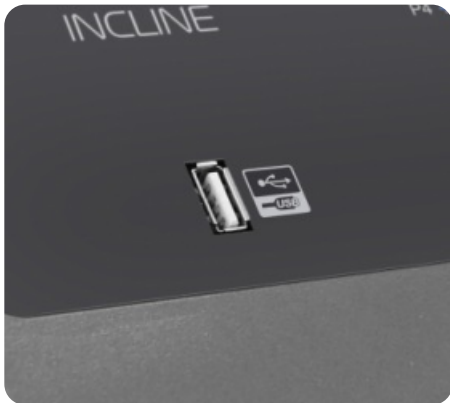
МУЛЬТИМЕДИЙНАЯ КОМПОНЕНТА
